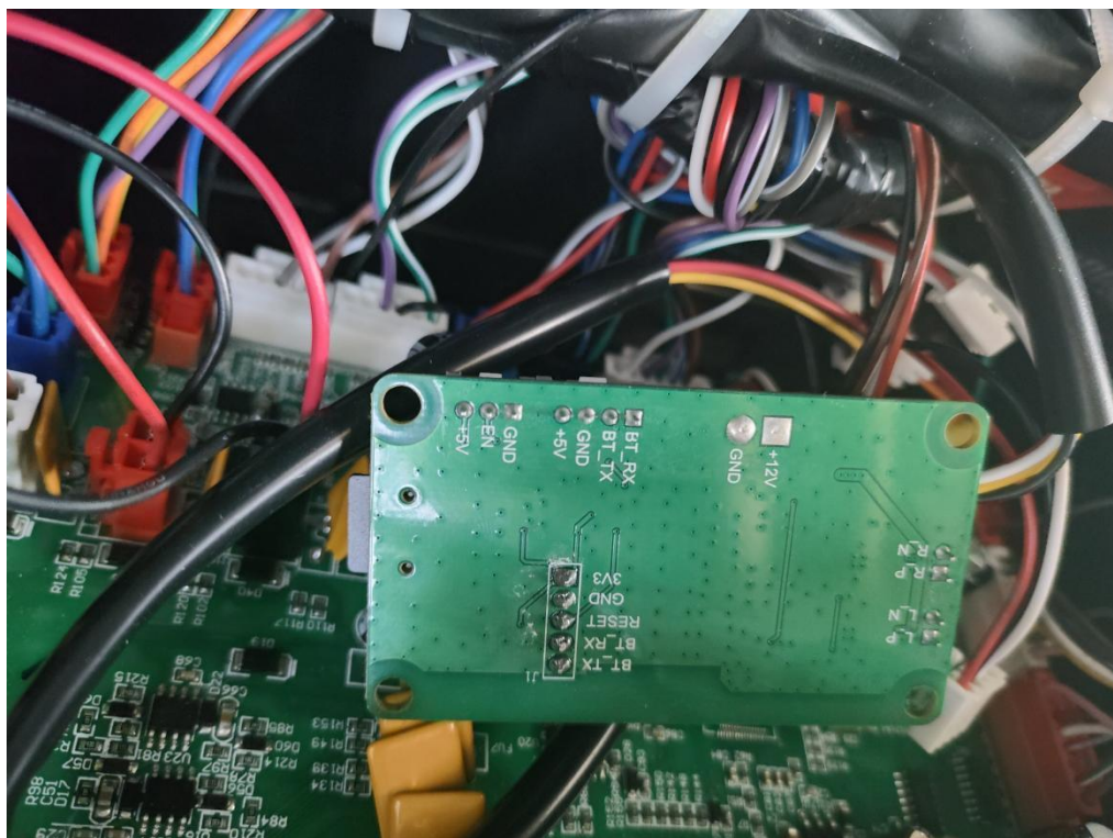
图片.14. PCB 视图
