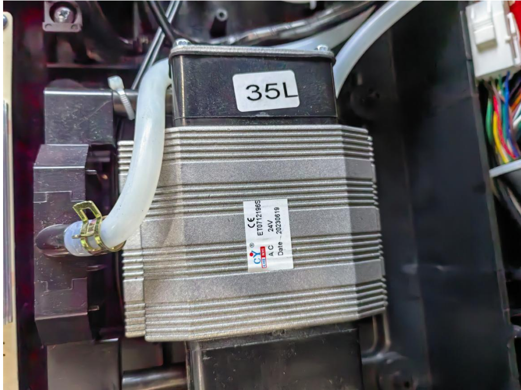
图片.17. 气泵视图
