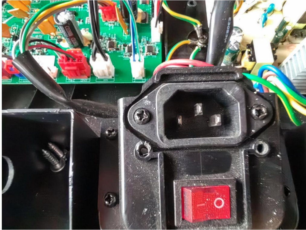
图片.7. 开关, 输入接口视图
